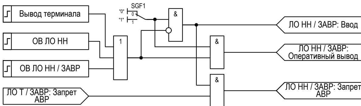
Рисунок 2.25 – Функциональная схема логики запрета АВР
